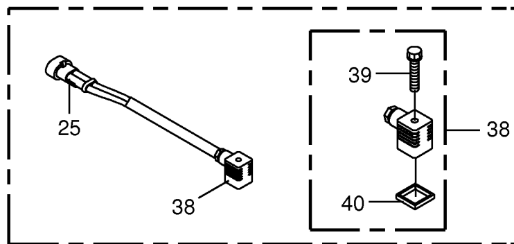
CAN Handbed-Metallortung
