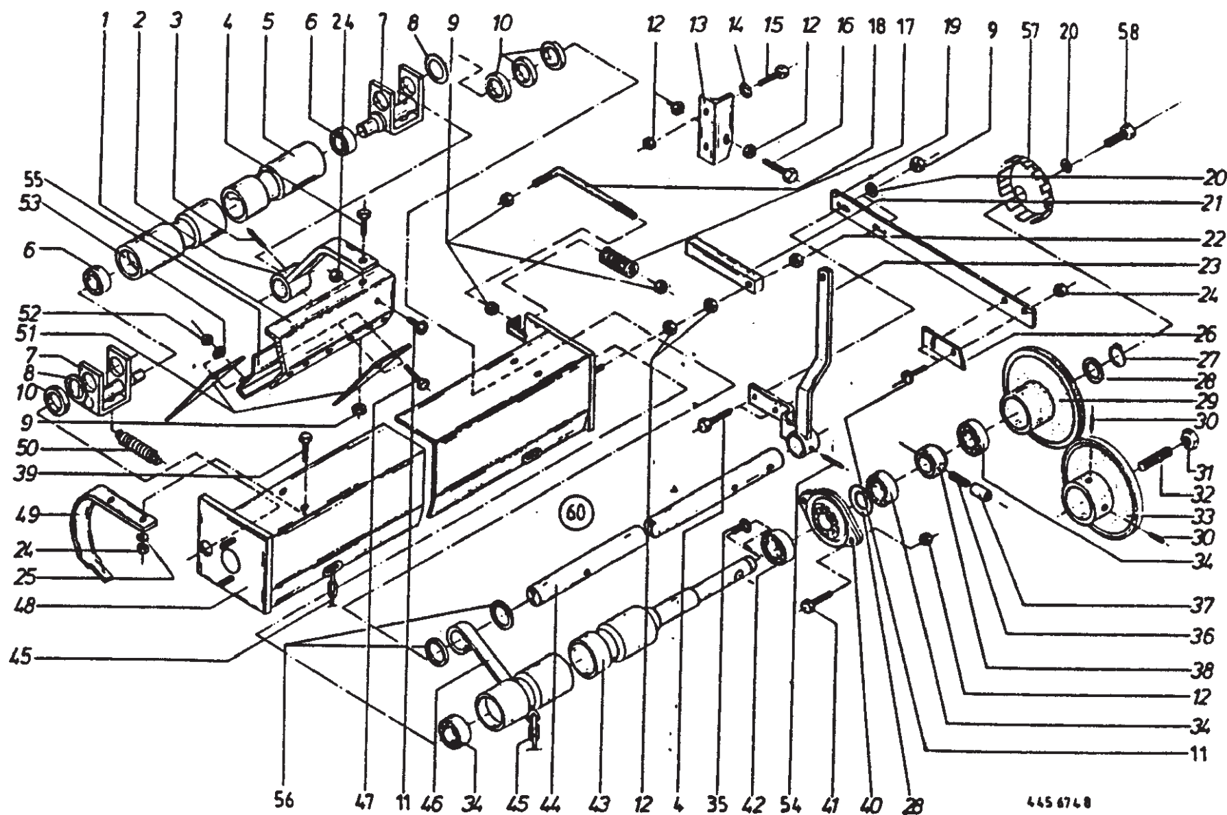
Net Wrap Unit
