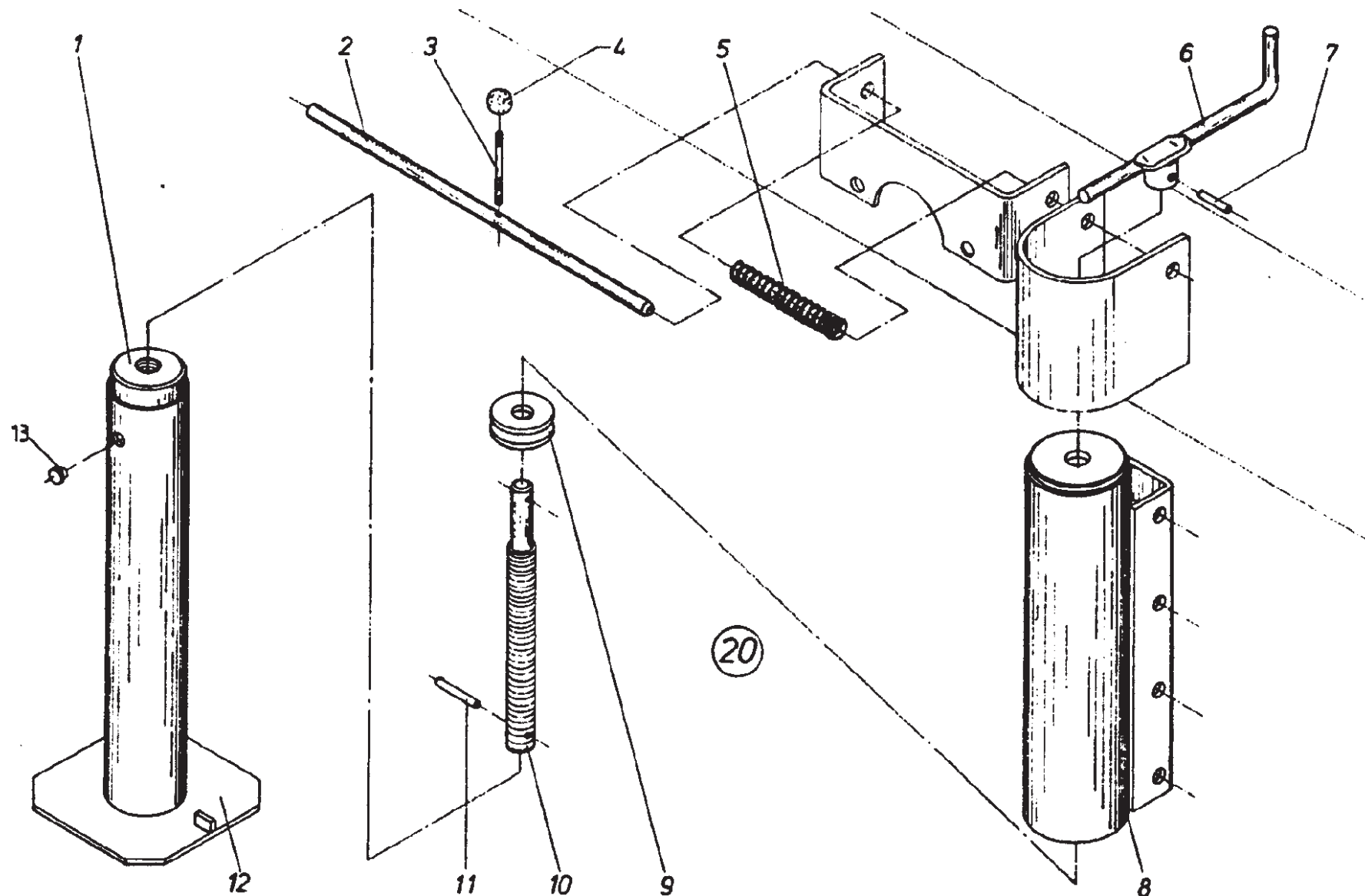
Jack Stand
