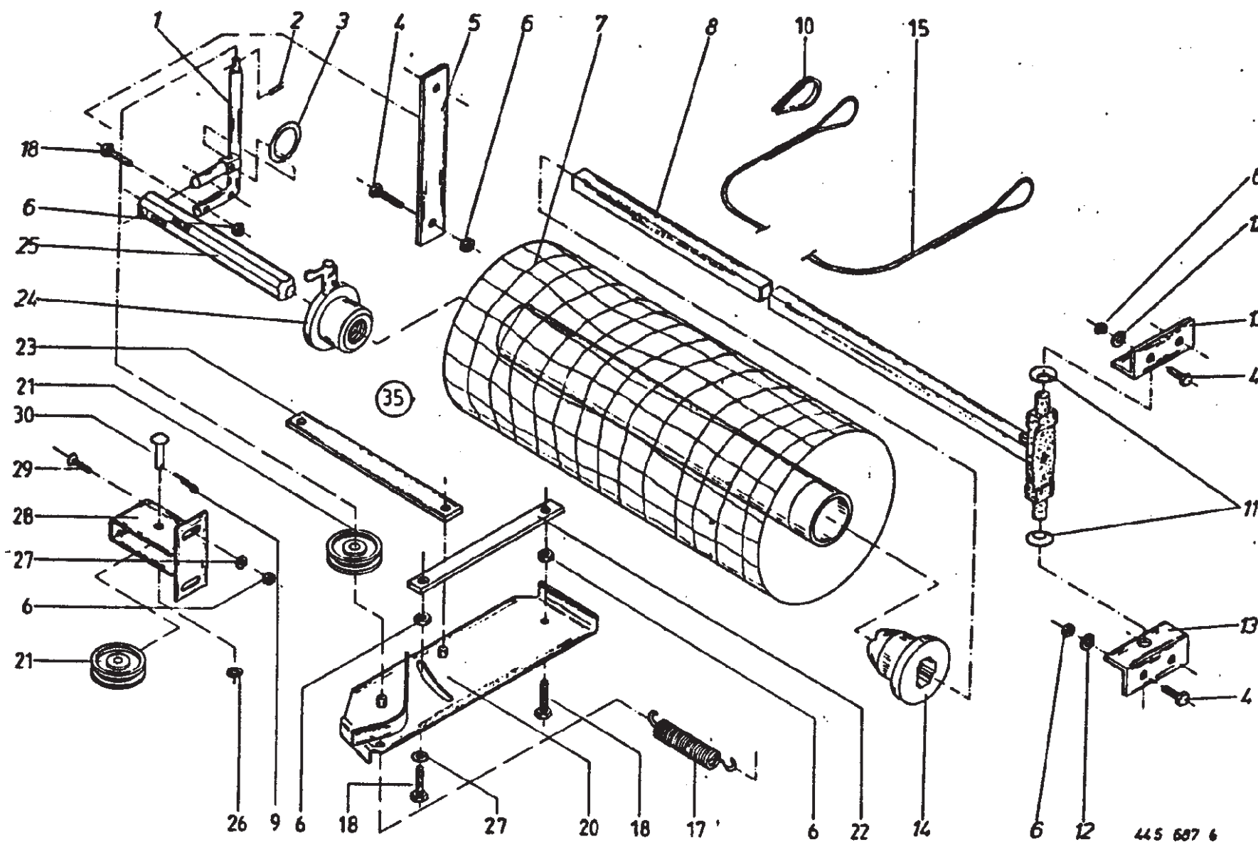
Net Wrap Brake
