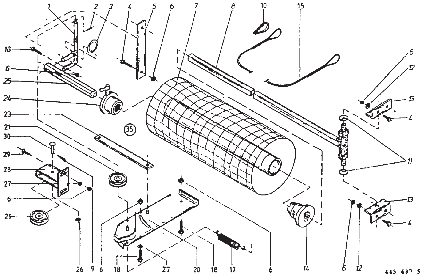
Net Wrap Brake
