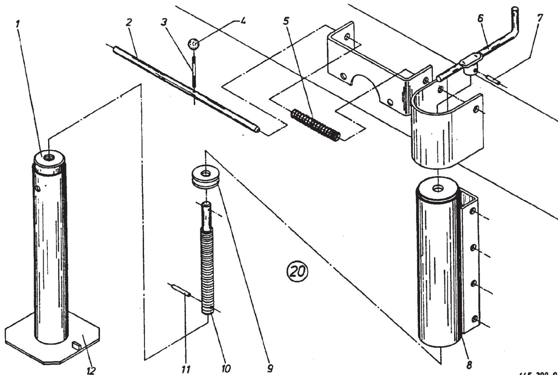
Jack Stand
