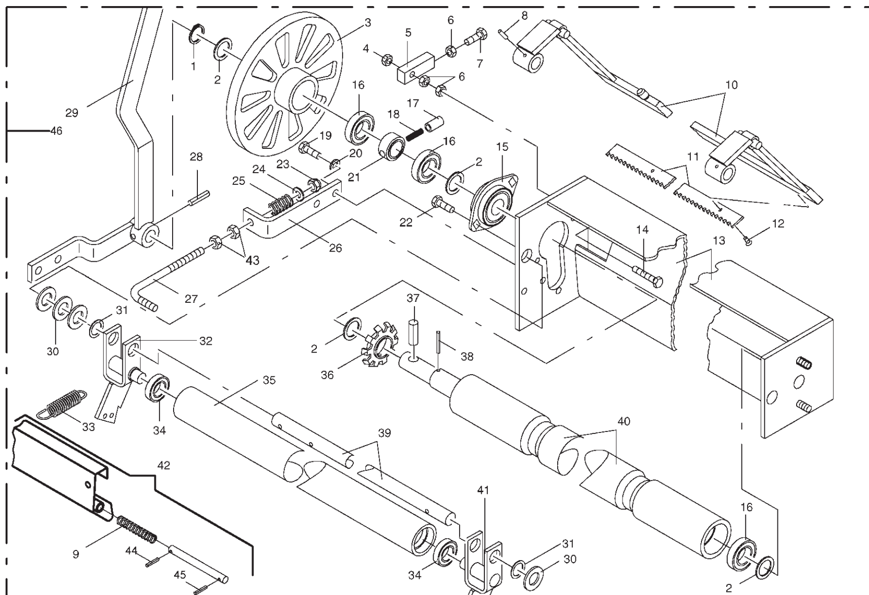
Net Wrap Unit
