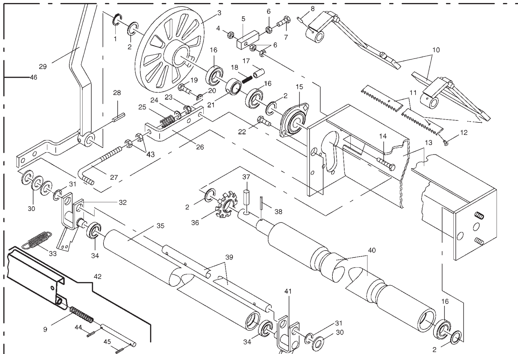
Net Wrap Unit
