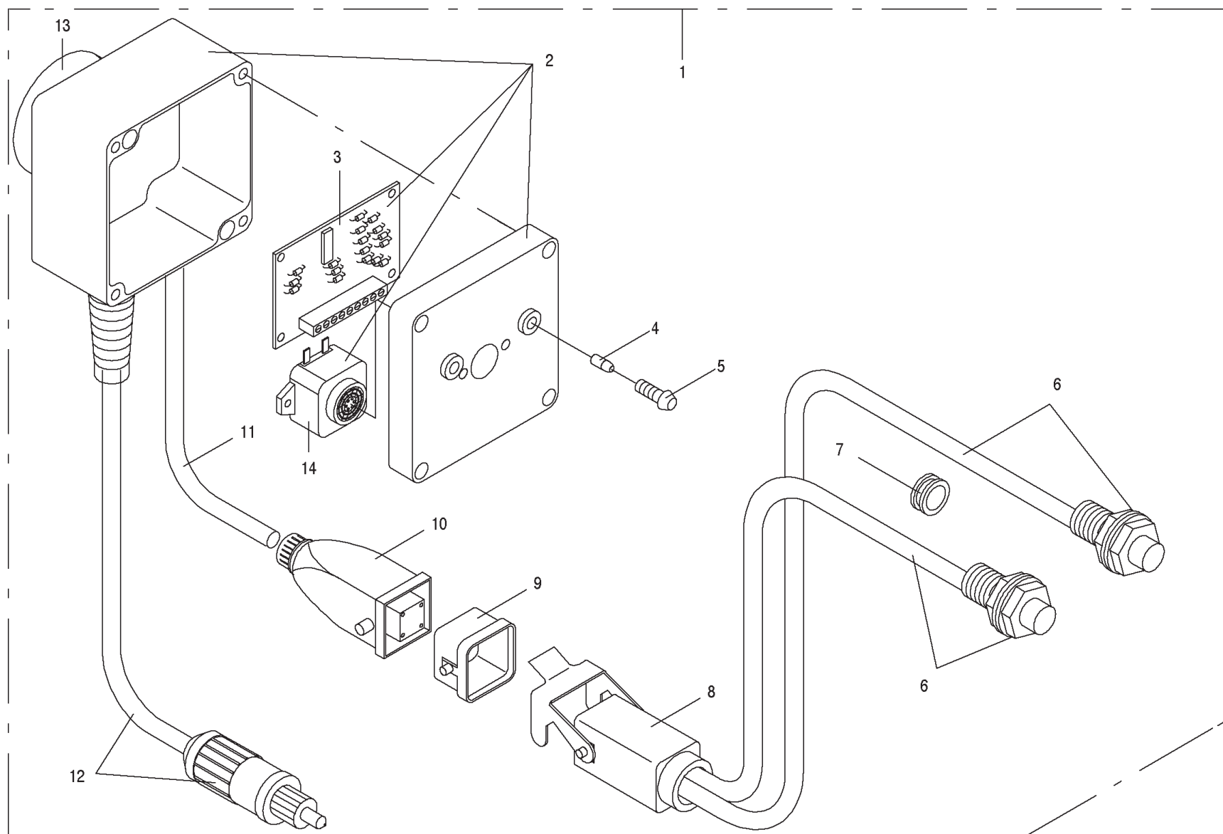
Optional Bale Monitor
